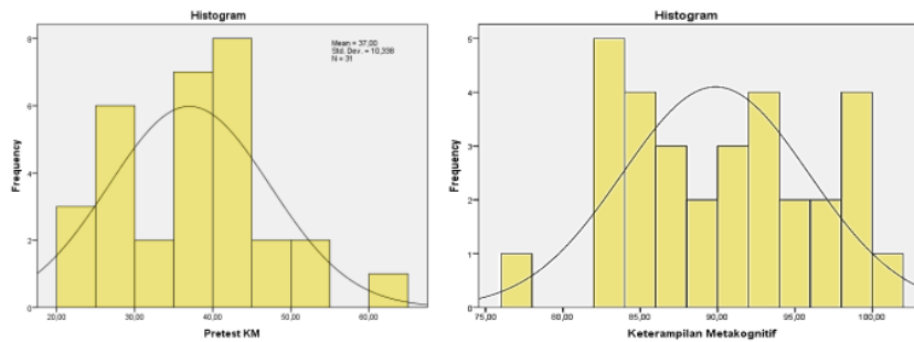
Gambar 1. Kurva data pretest-posttest keterampilan metakognitif berdistribusi normal
